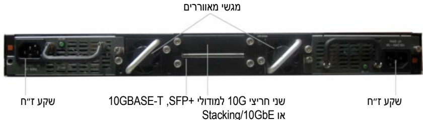
איור 10-1. PC7048R – לוח אחורי
